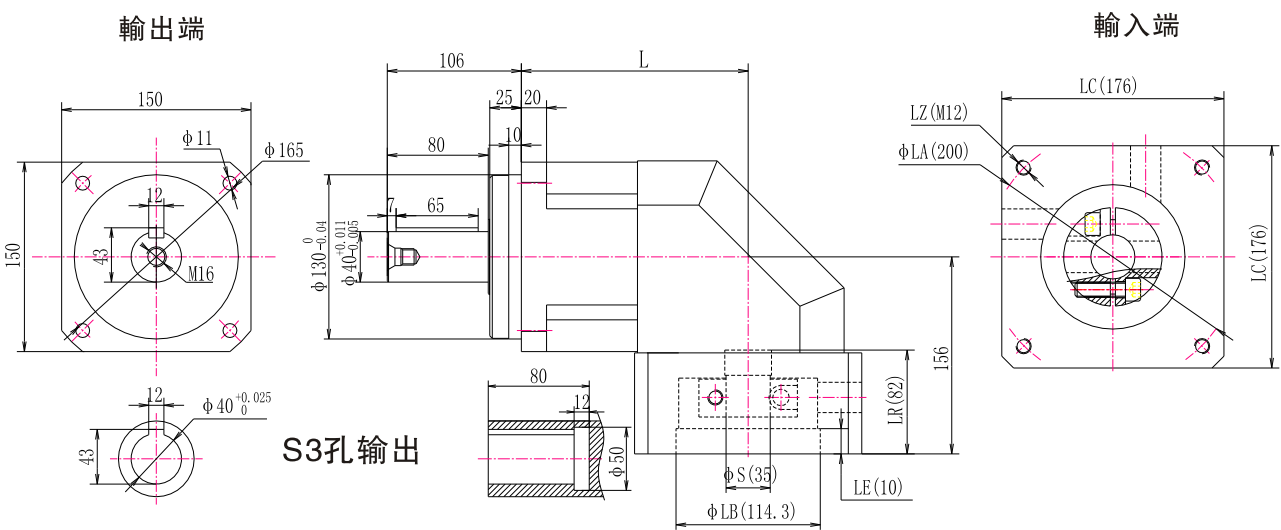
USR142外形图
