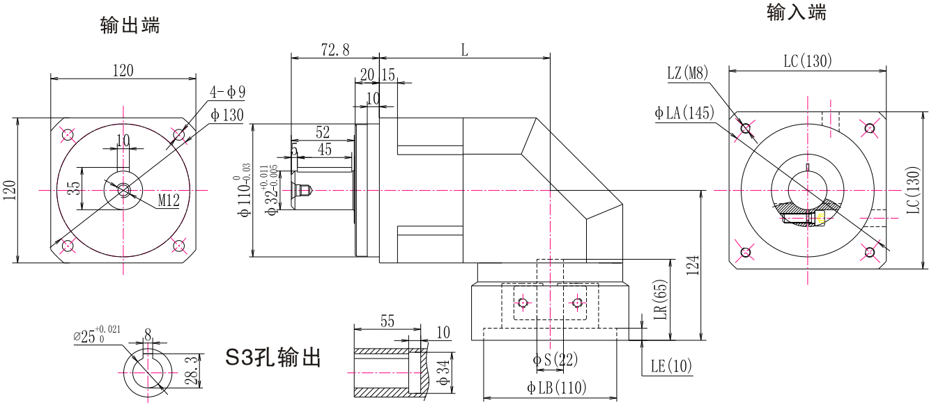
USR115外形图
